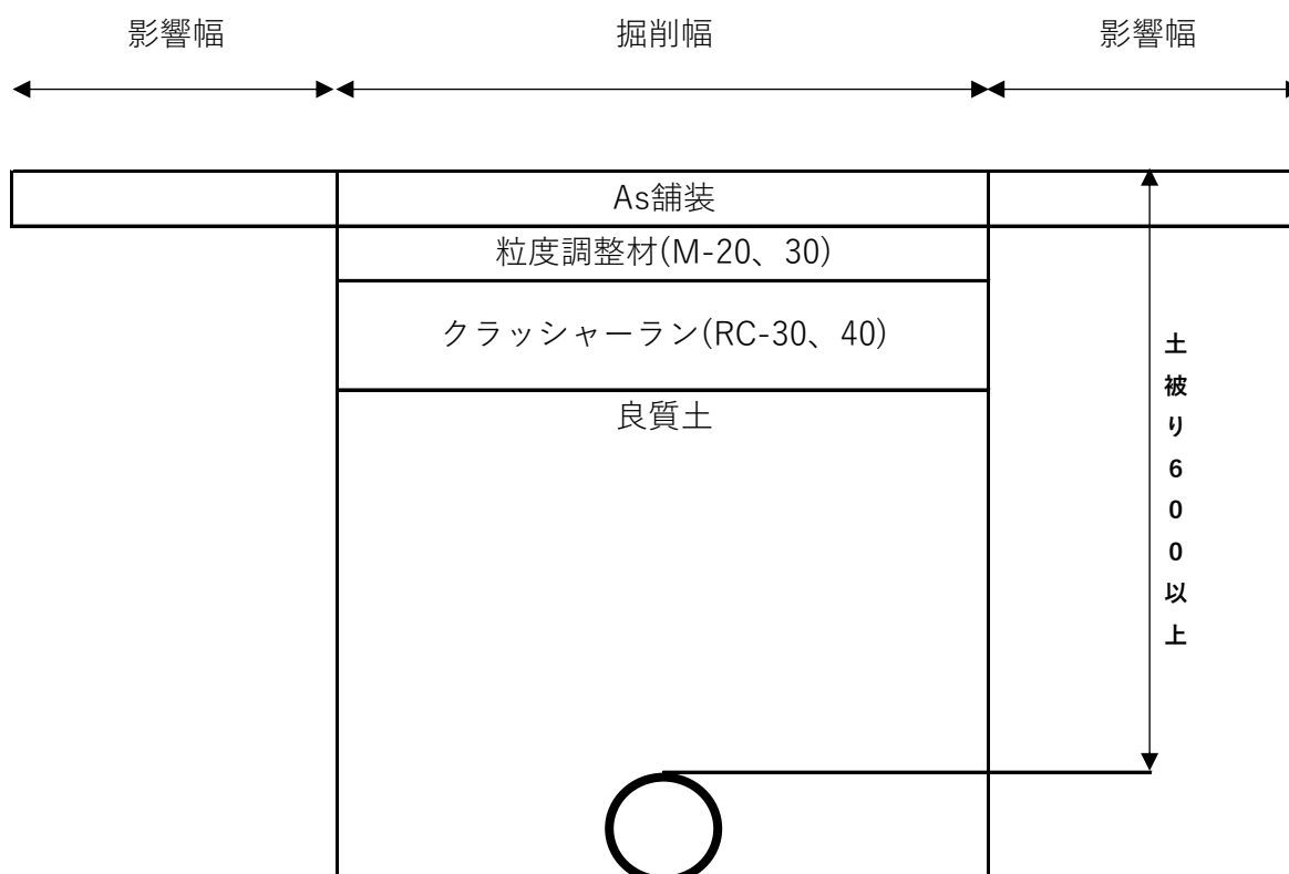
復旧断面図
