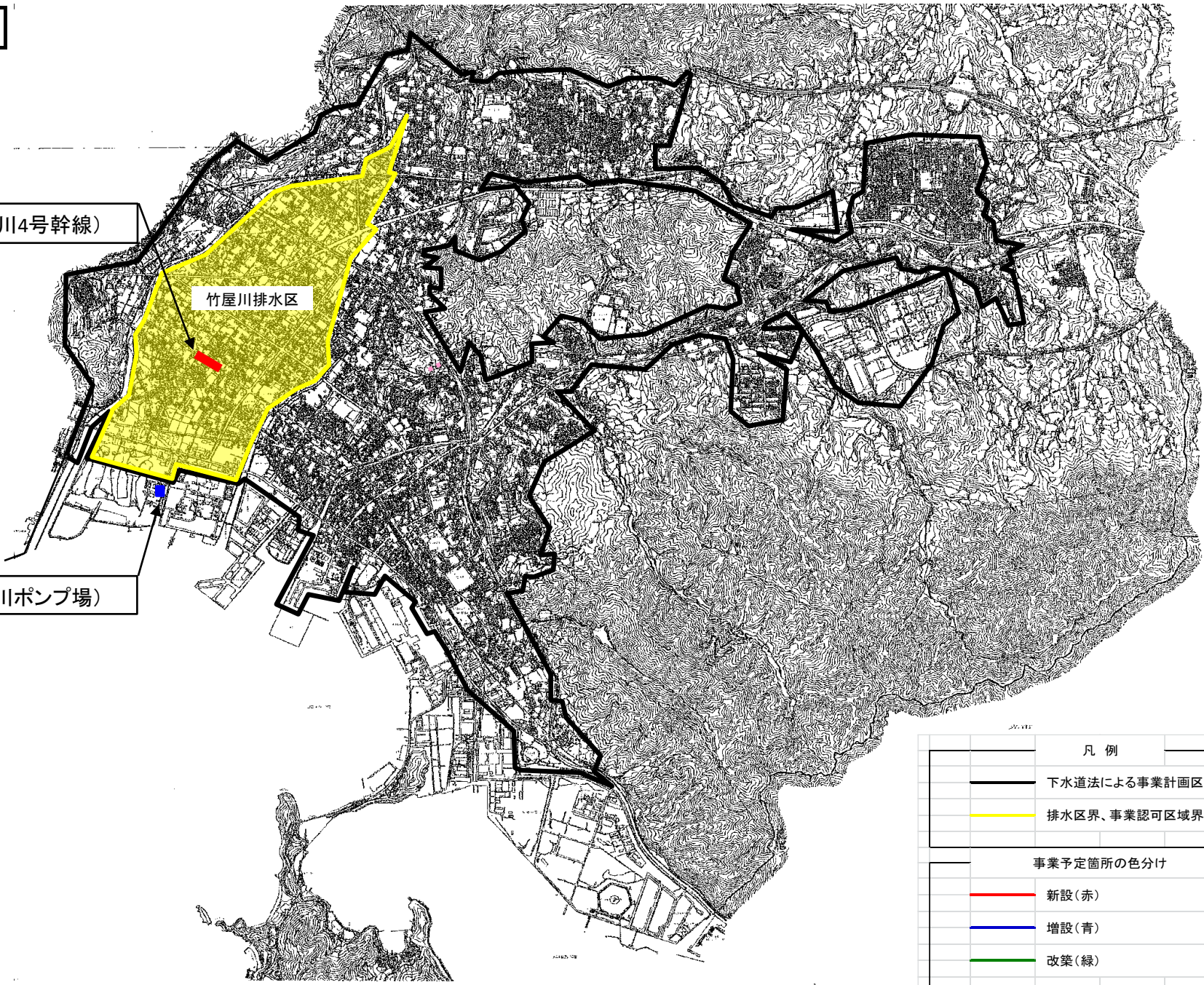
竹屋川排水区計画図
