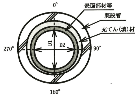
図 参 6-7-1 仕上がり内径を測定する位置
