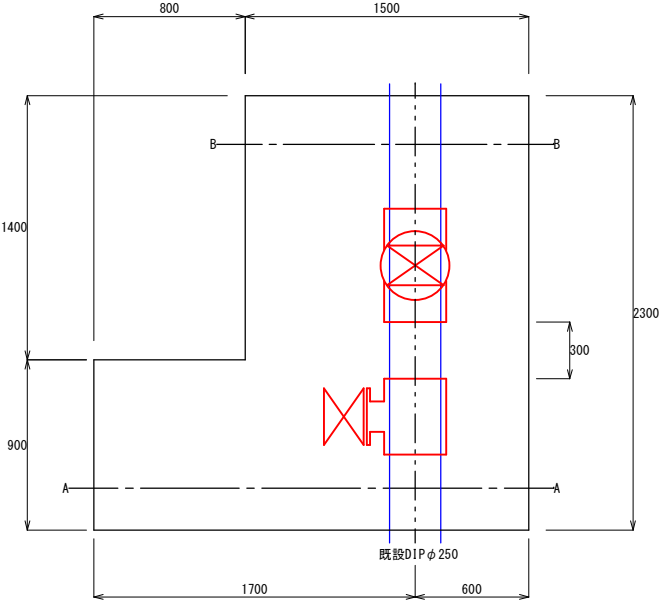
掘削平面
