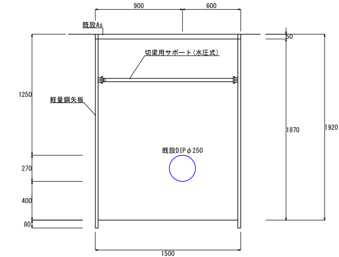
復旧断面
