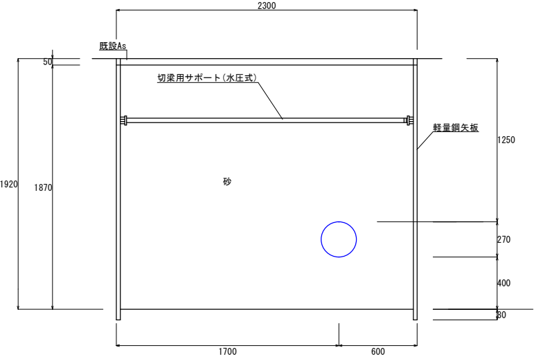
復旧断面
