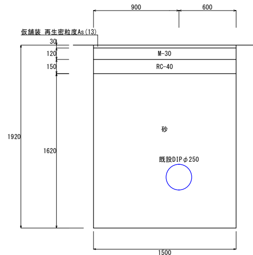
復旧断面
