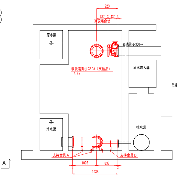
D-D断面図
