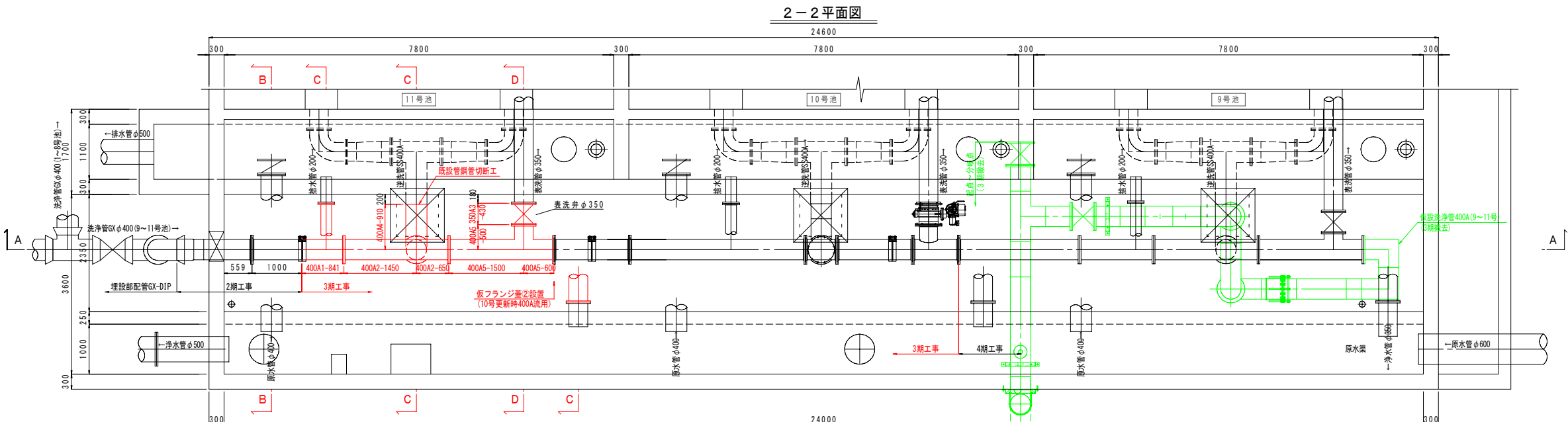
1-1平面図
