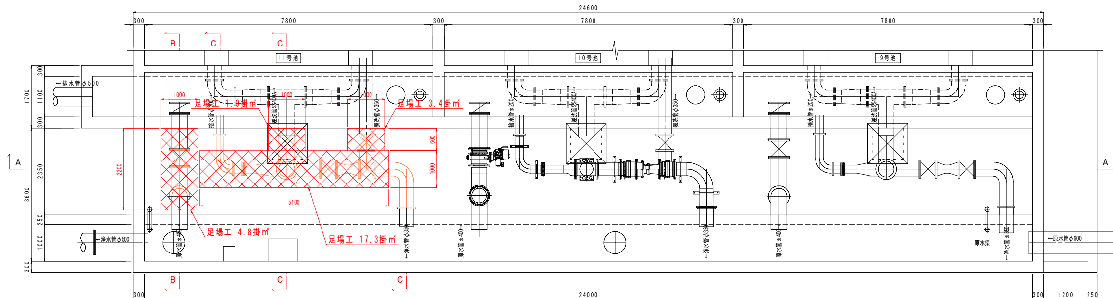
1-1 平面图
