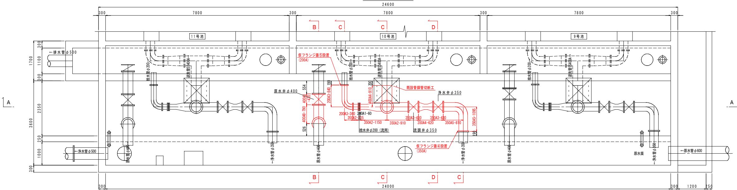
1-1平面図
