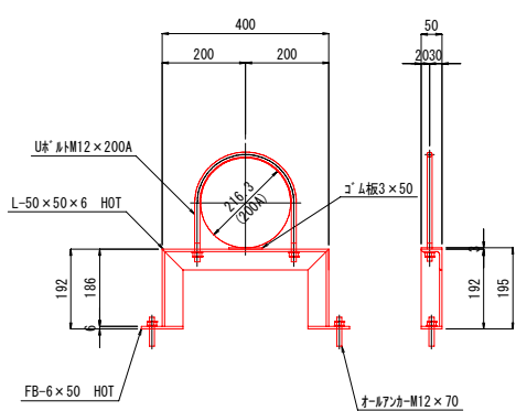
断面図
