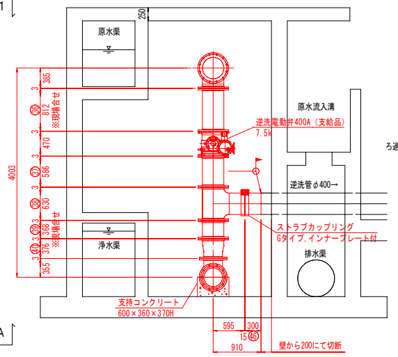
D-D断面図
