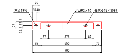
平面図
