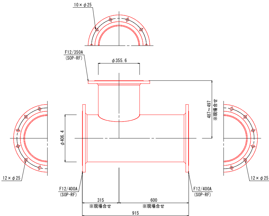
管番号 ③②: 3F T字管 数量: 2本 10号: 1本 11号: 1本
