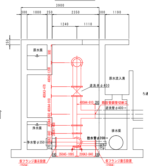
D-D断面図
