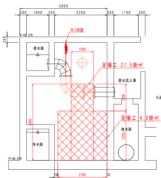
B-B断面図
