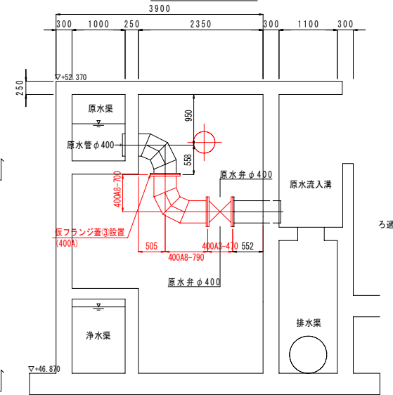
C-C断面図
