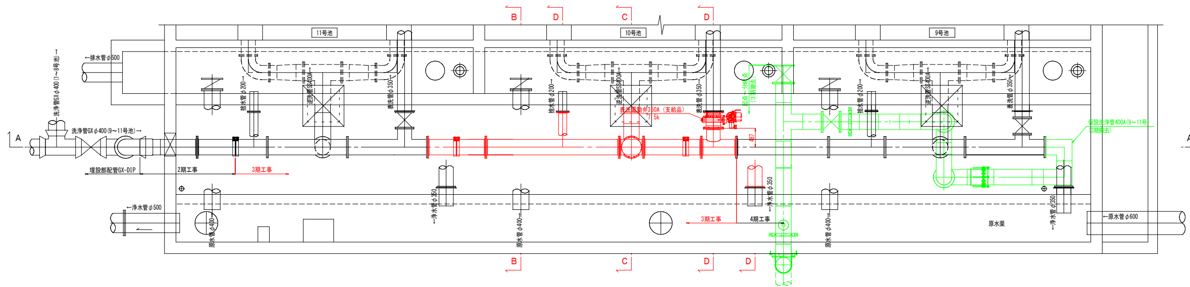
1-1平面図
