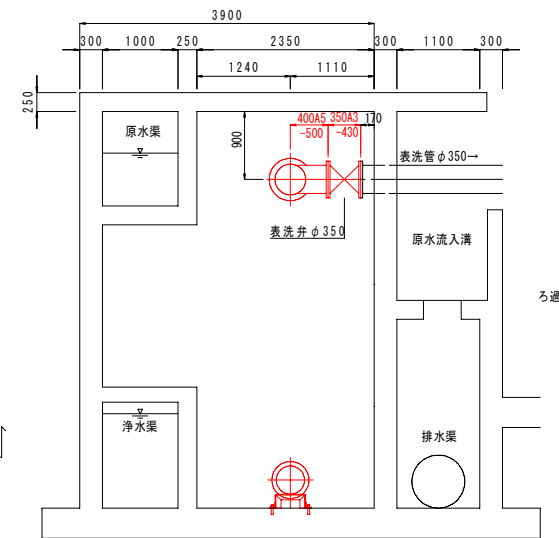
D-D断面図
