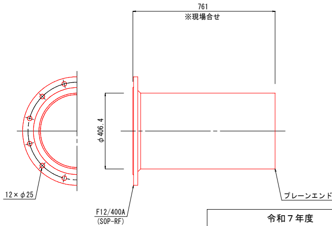
管番号 ③④: 2F 直管 数量: 1本 10号: 1本
