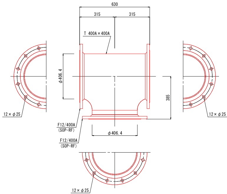
管番号 ③②: 3F T字管 数量: 2本 10号: 1本 11号: 1本
