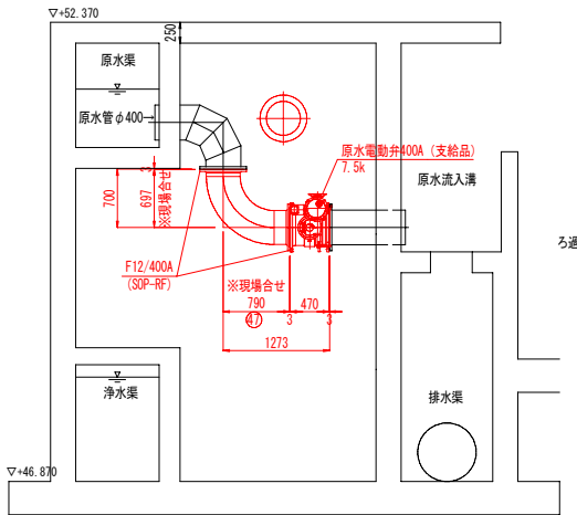
C-C断面図
