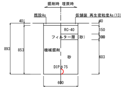
土工② (1級市道歩道一般車両乗入部)
