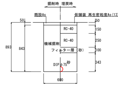
土工③ (1級市道歩道大型車両乗入部)
