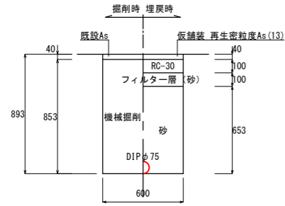
土工① (1級市道歩道一般部)
