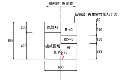
土工④ (1級市道車道部)
