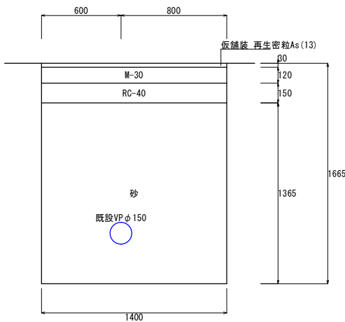
復旧断面
