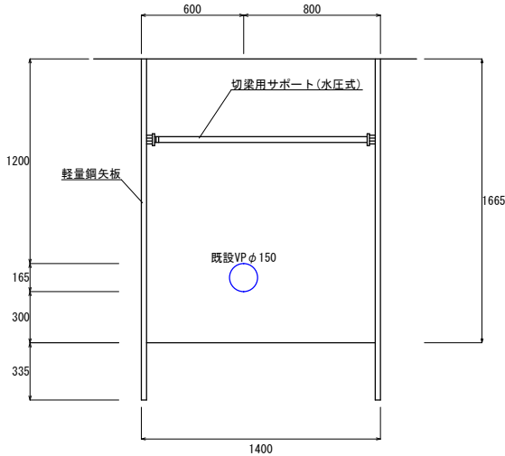
復旧断面
