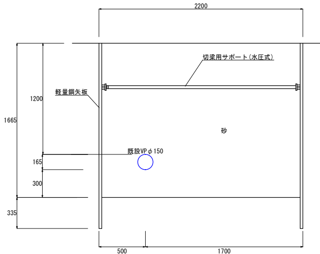
復旧断面
