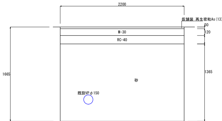
復旧断面
