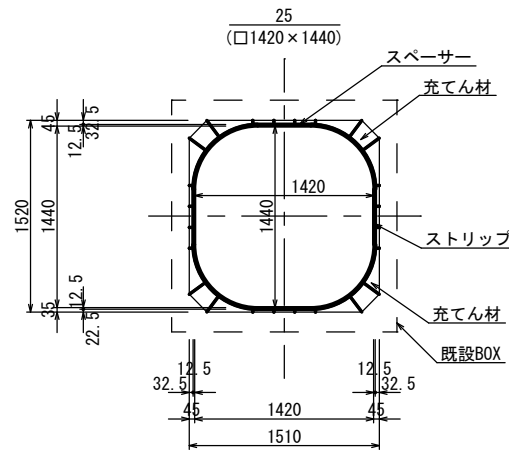
更生管標準断面図 S=1:30 (複合管)
