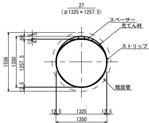
更生管標準断面図 S=1:30 (複合管)
