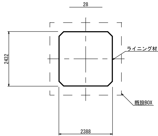
修繕工標準断面図 S=1:50 (修繕工法)
