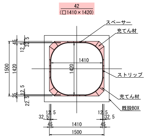
更生管標準断面図 S=1:30 (複合管)
