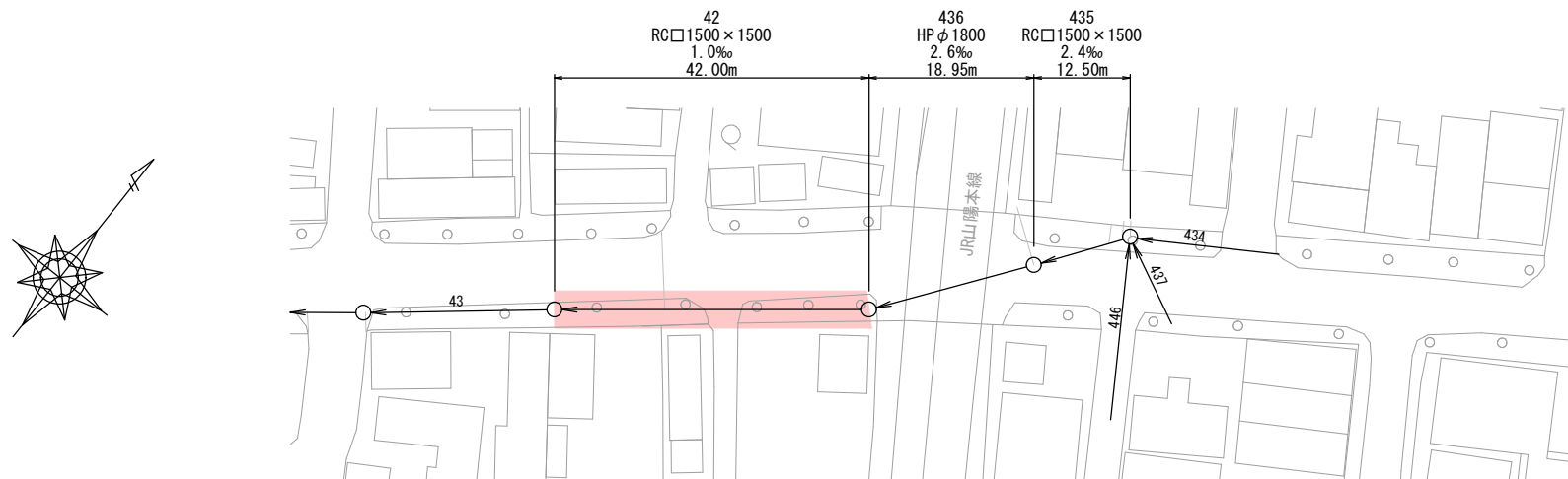
平面図 S=1:500
