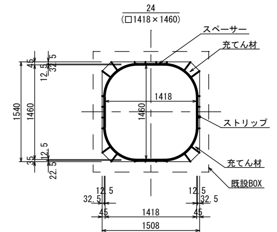
更生管標準断面図 S=1:30 (複合管)
